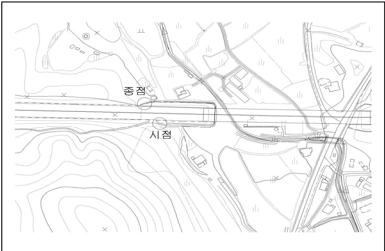
&lt;그림 1.3.1&gt; 설계도면 선형과 금회 실측 값 비교
