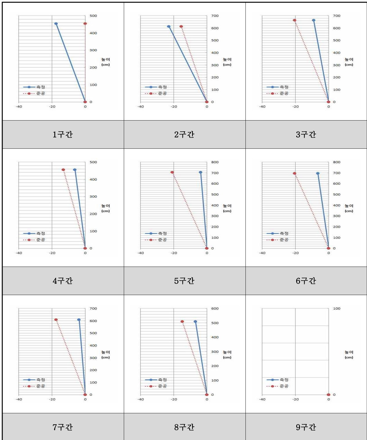
&lt;그림 1.3.2&gt; 계획선형 오차 측정결과
